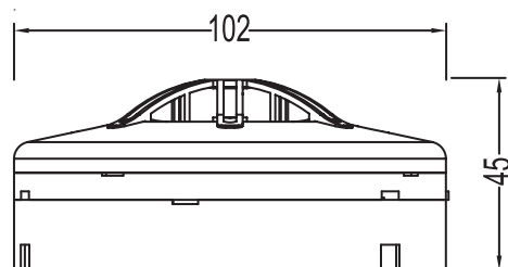
尺寸圖
