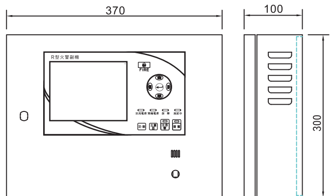
尺寸圖
