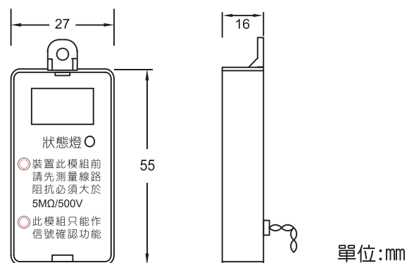
尺寸圖
