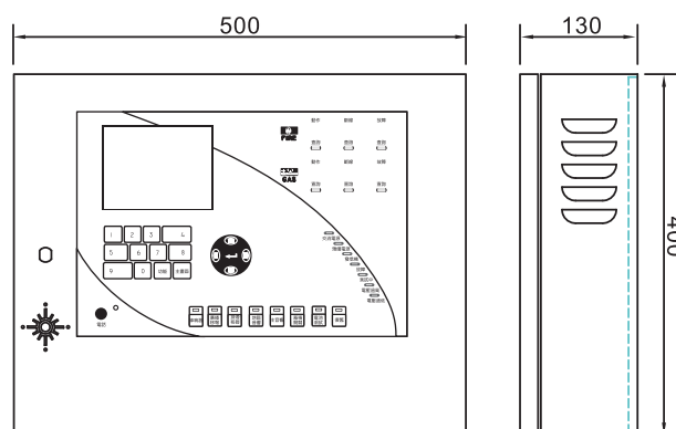
尺寸圖
