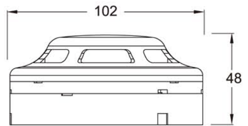
尺寸圖
