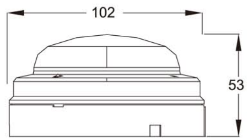
尺寸圖
