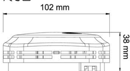
尺寸圖
