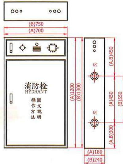
露出型示意圖
