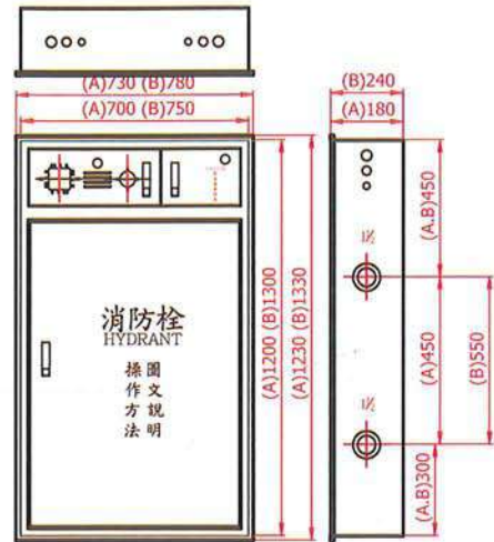
埋入型含緊急電源示意圖
